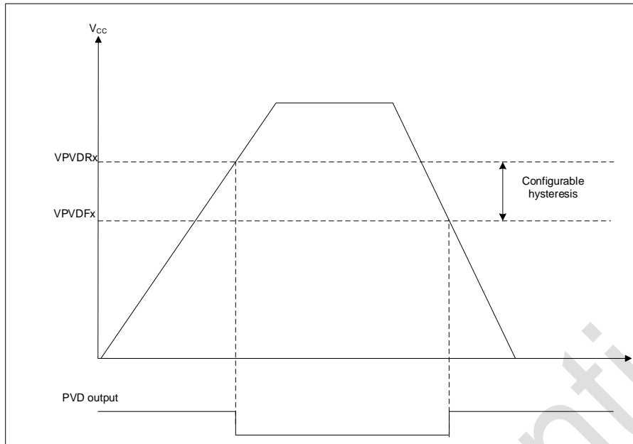
图 2-3 PVD 阈值
