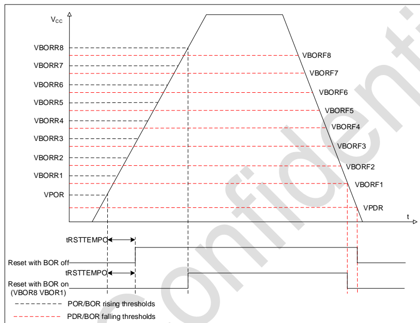
图 2-2 POR/PDR/BOR 阈值
