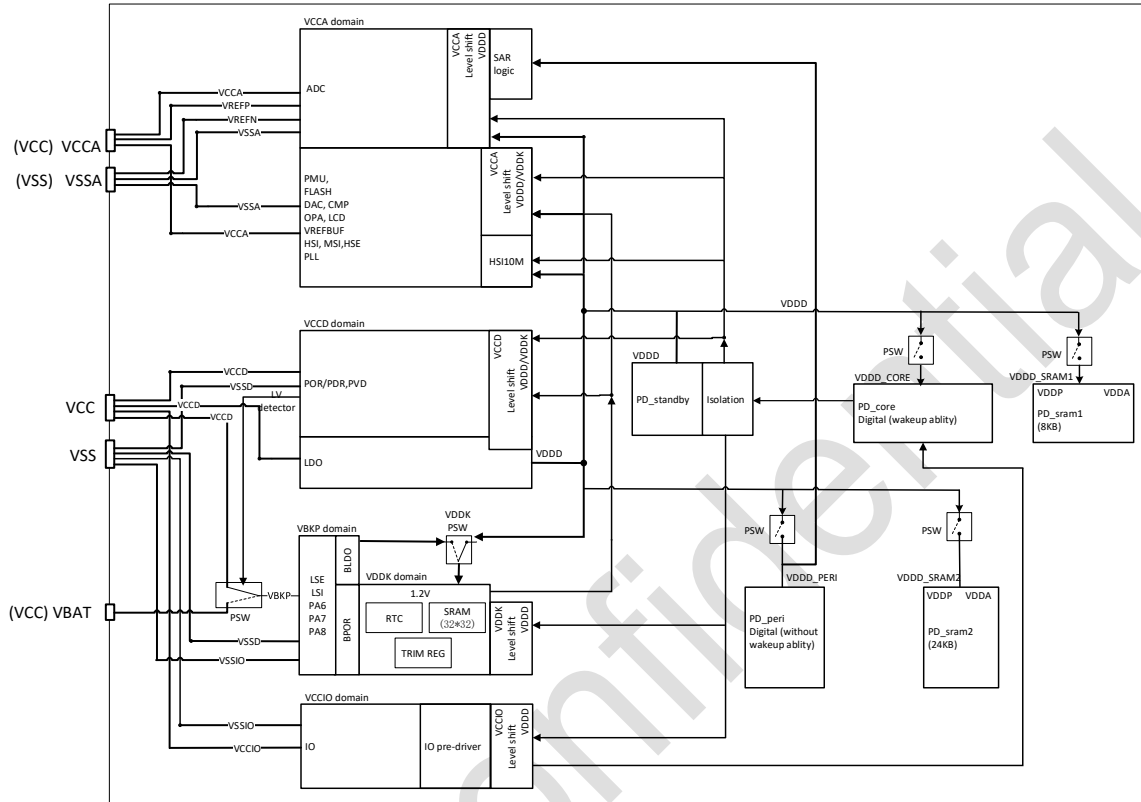
图 2-2 电源框图
