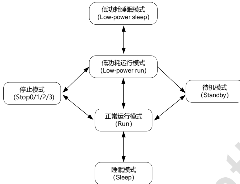
图 2-4 功耗状态转换图
